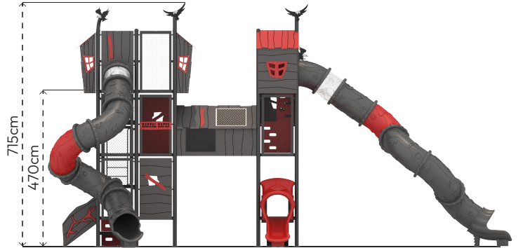
Ön Görünüş
