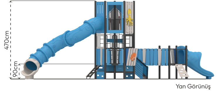
Yan Görünüş
