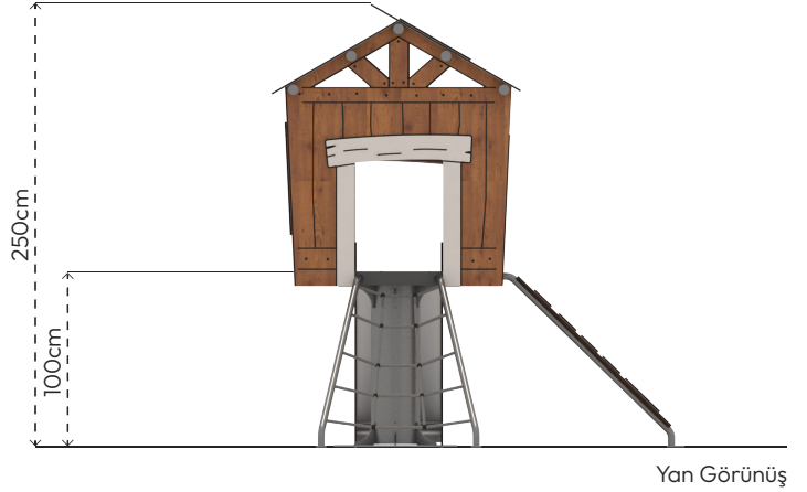
Yan Görünüş
