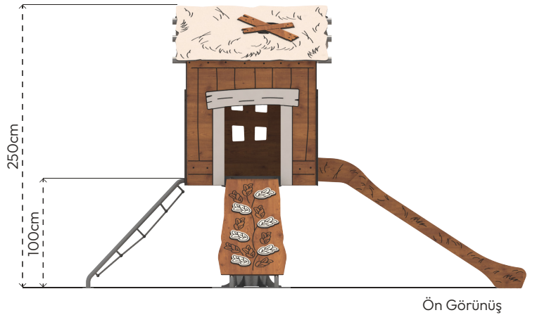
Ön Görünüş
