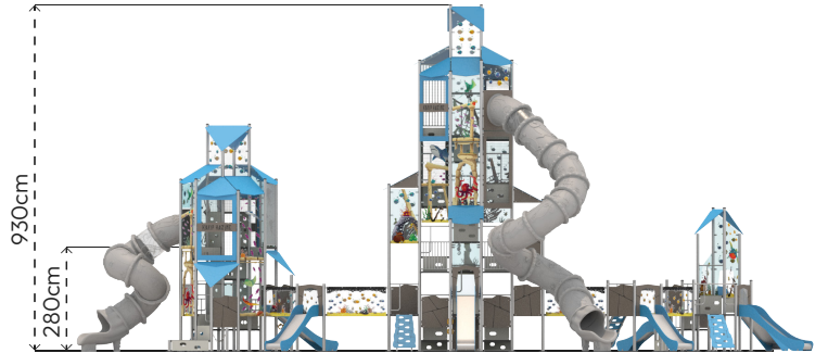
Ön Görünüş
