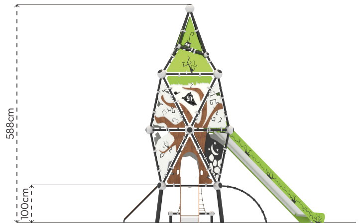
Ön Görünüş
