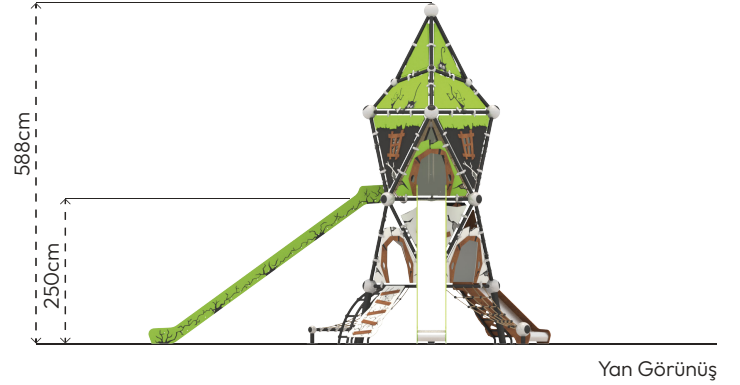
Yan Görünüş
