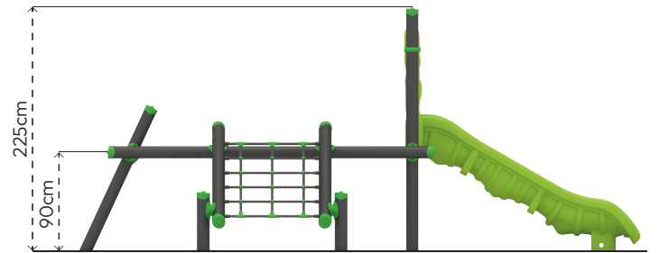
Ön Görünüş
