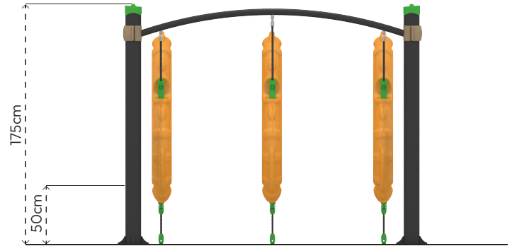
Ön Görünüş
