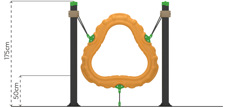
Yan Görünüş
