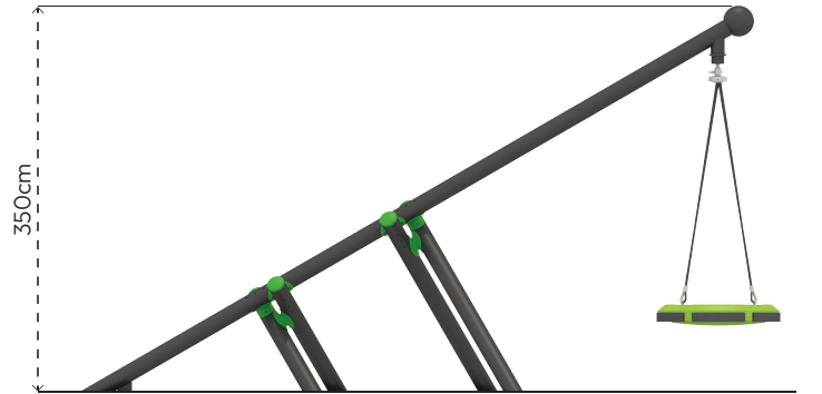
Ön Görünüş
