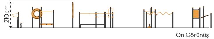
Ön Görünüş
