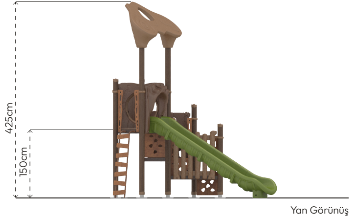
Yan Görünüş
