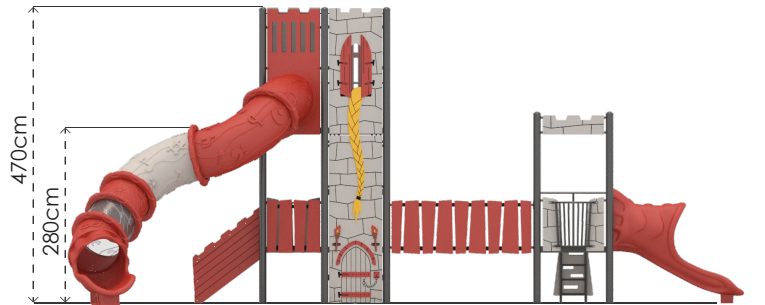
Ön Görünüş
