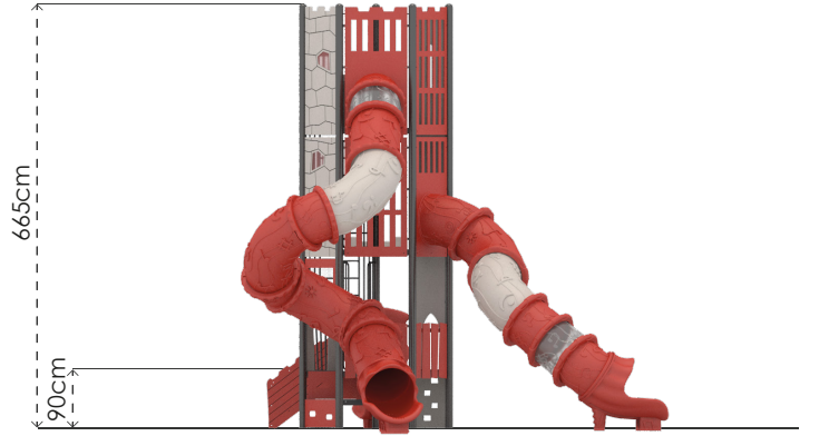
Yan Görünüş
