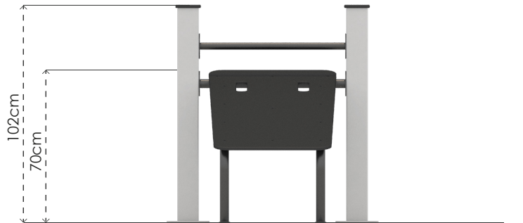
Ön Görünüş
