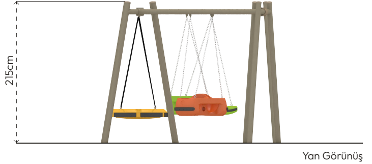
Yan Görünüş
