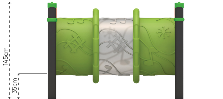
Ön Görünüş
