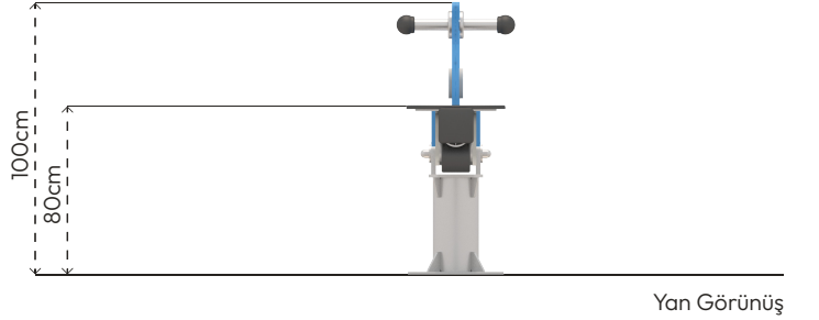
Yan Görünüş
