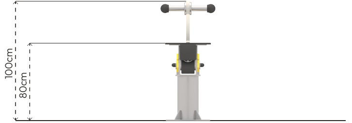
Yan Görünüş
