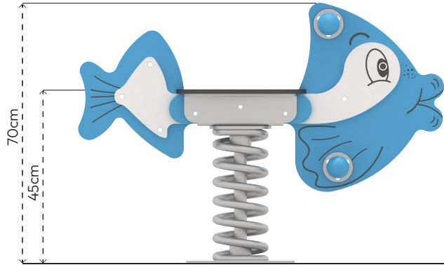
Ön Görünüş
