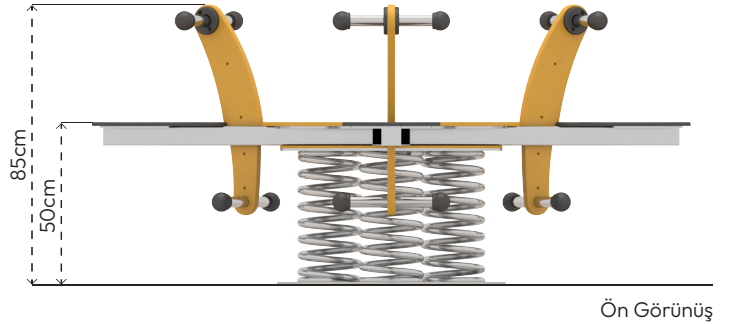
Ön Görünüş
